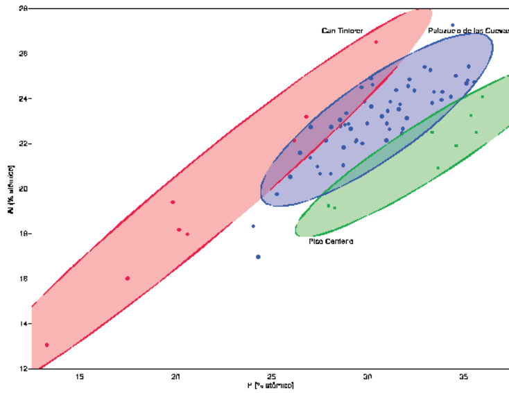
Figura 2 – Composições das contas variscite de VNSP. Elipses de confiança a 90% para os rácios P/Al atómicos de cada fonte.
