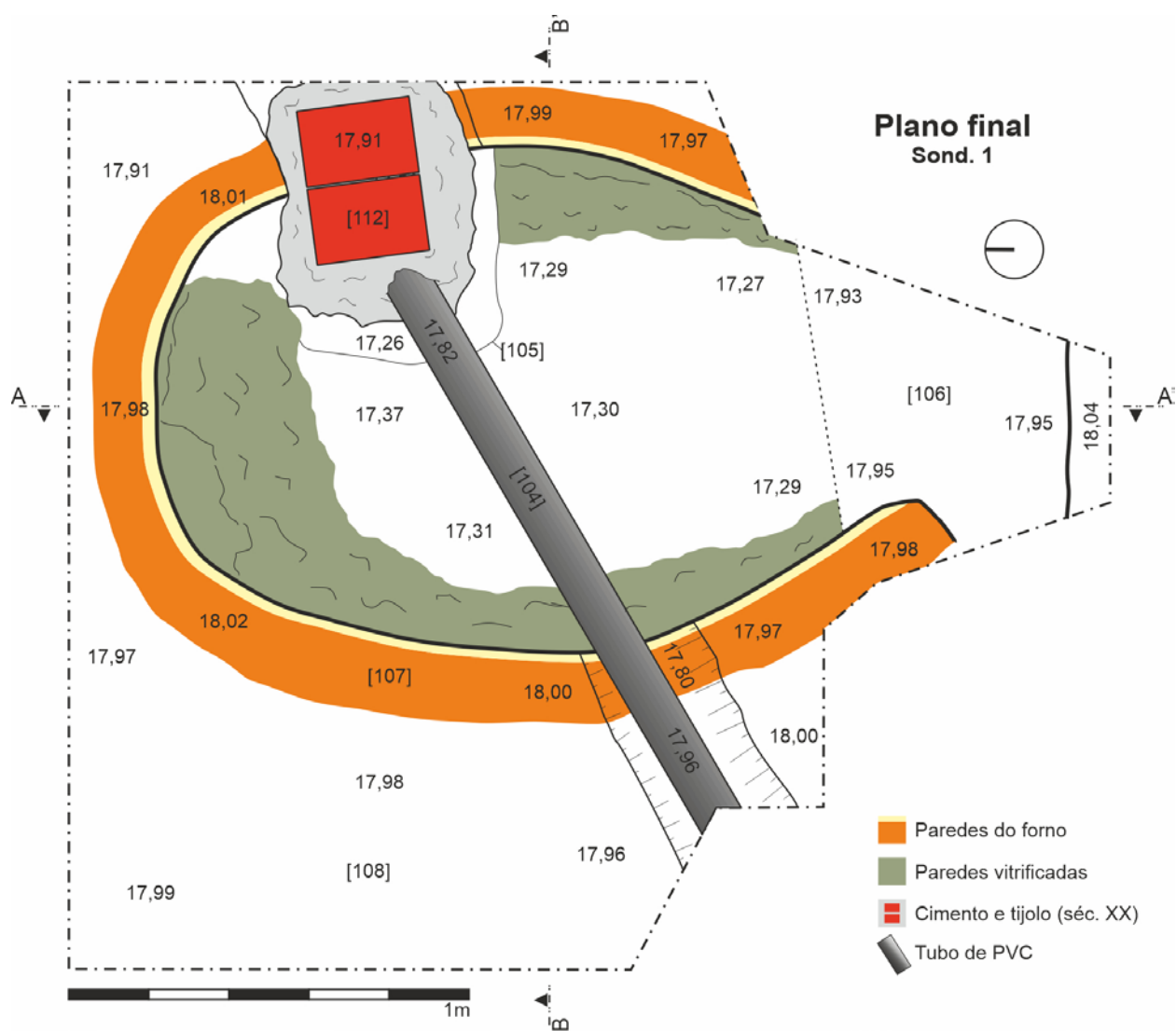
Figura 2 – Plano final do forno.
