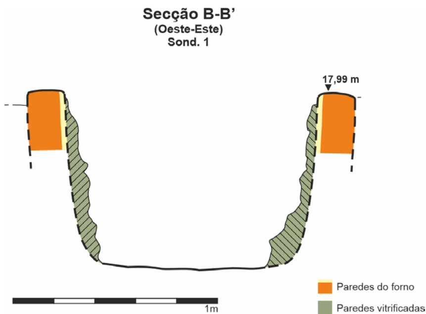
Figura 4 -Secção transversal da estrutura de combustão.
