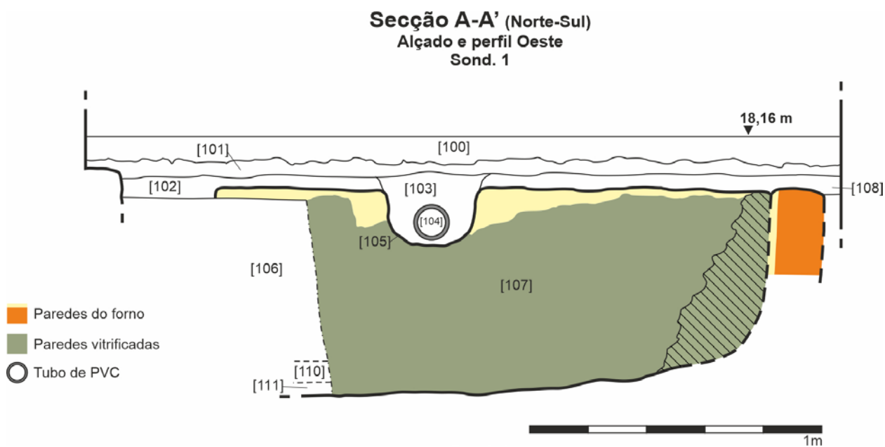
Figura 3 -Secção longitudinal e alçado do interior da estrutura de combustão.
