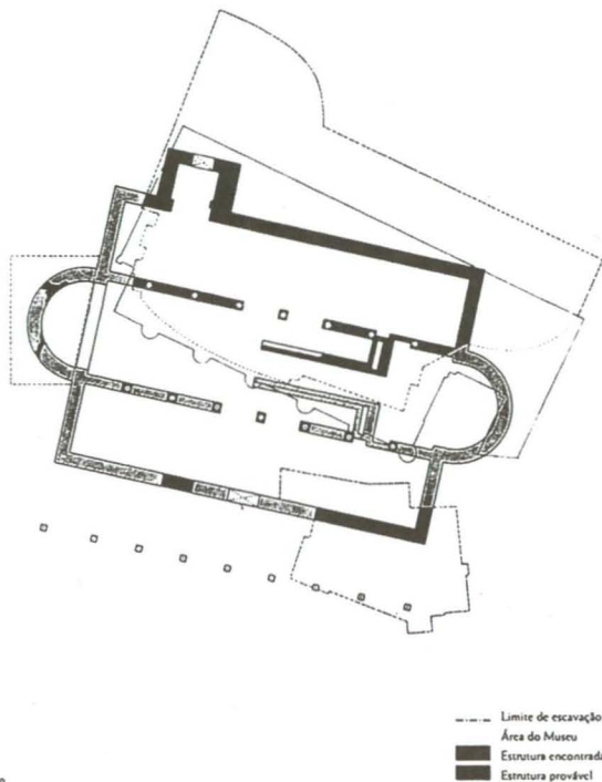
5c. Planimetria da basílica paleocristã de Mértola, segundo Cláudio Torres e Santiago Macias (1993:Fig.8). Esc.1:500
